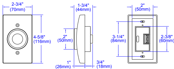
Montaje empotrado
